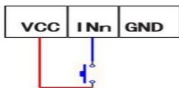
干触点接法
