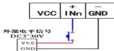
湿触点接法
